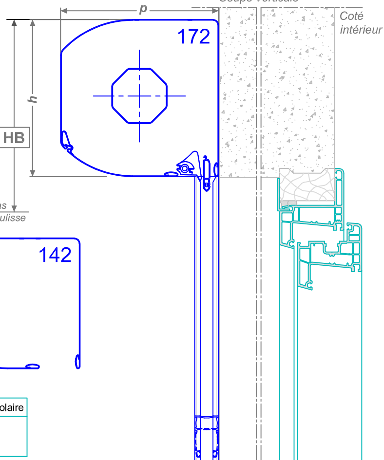
Coupe verticale
