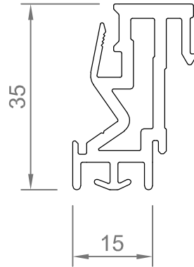
Elargisseur EL
