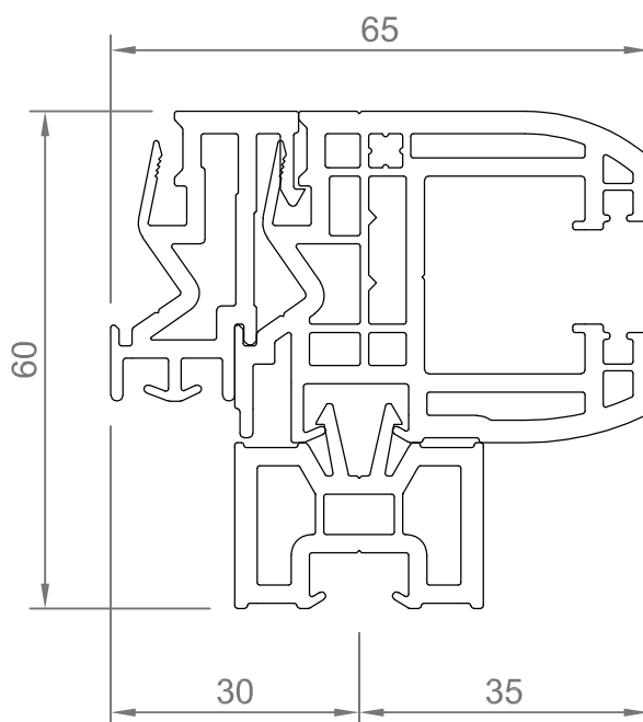
Coulisse U6 avec élargisseur EL
