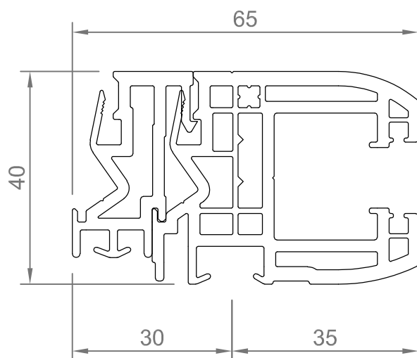
Coulisse U4 avec élargisseur EL
